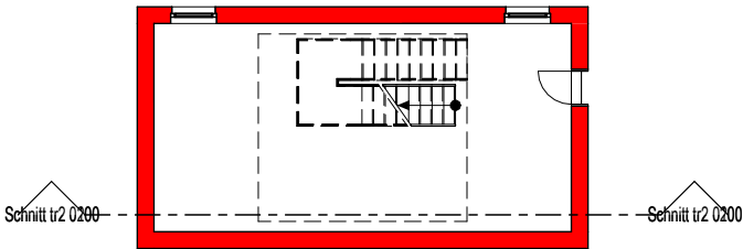
Erdgeschoss M 1 : 200
