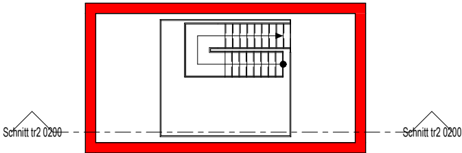
1. Obergeschoss M 1 : 200
