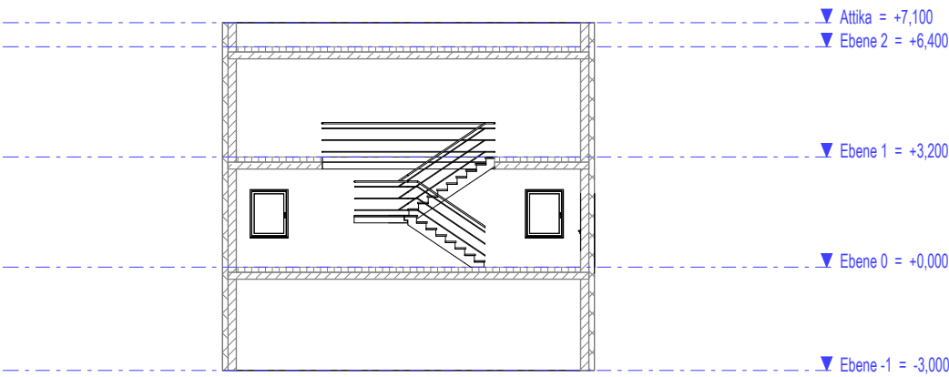
Schnitt tr2 0200 M 1 : 200
