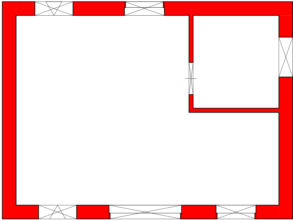
Grundriss; Detaillierungsgrad: grob M 1 : 50
