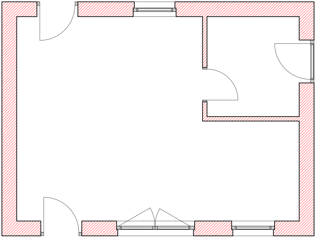
Grundriss; Detaillierungsgrad: mittel M 1 : 50
