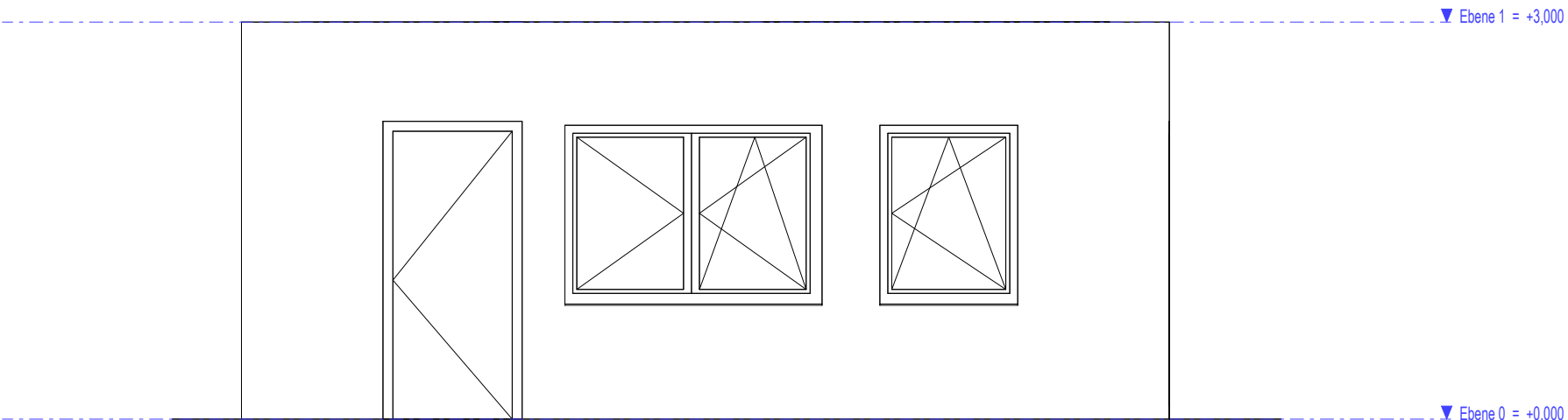
Süd Detaillierungsgrad mittel R M 1 : 50
