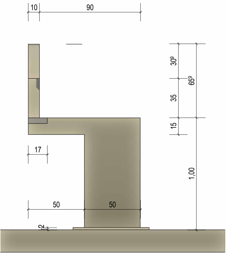
Ansicht von vorn M 1:20
