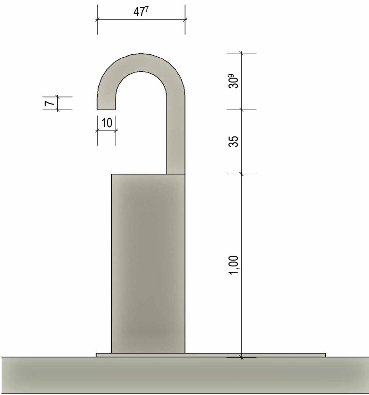
Ansicht von rechts M 1:20
