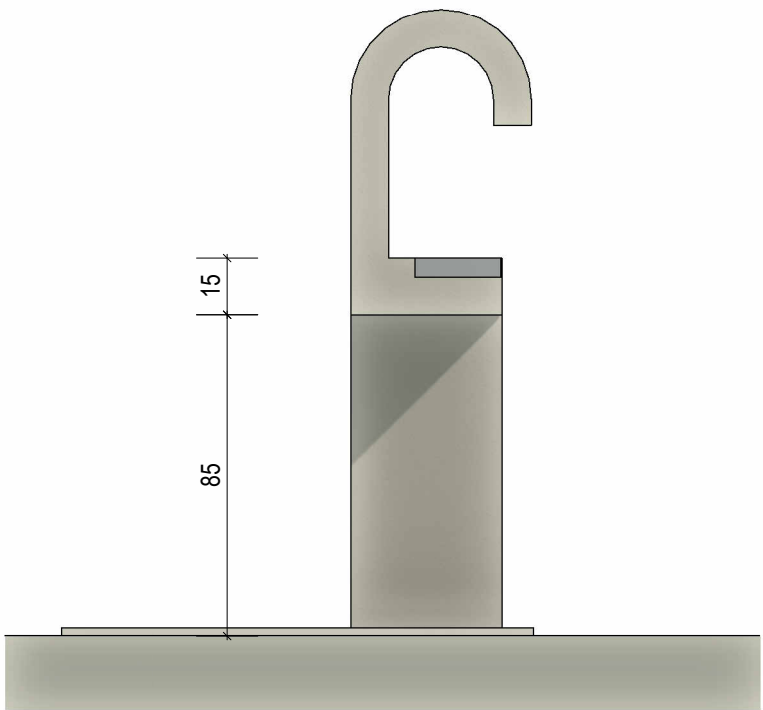
Ansicht von links M 1:20
